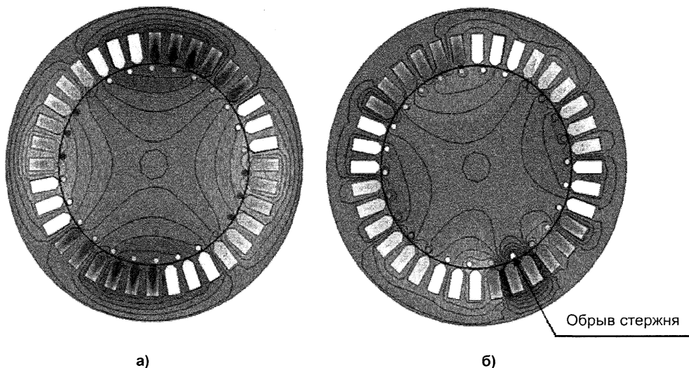
Рис. 3. Мгновенная картина магнитного поля в поперечном сечении: а) исправный АД, б) АД со сломанным стержнем ротора
