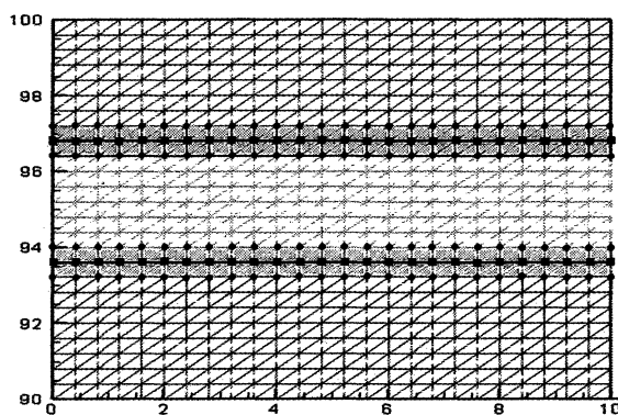
Рис. 4. Декомпозиция с теневыми границами
