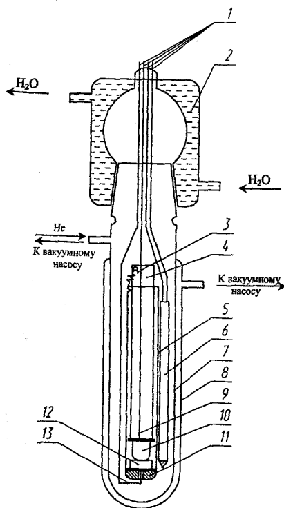
Рис. 2. Схема гальванической ячейки
