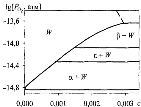
Рис. 8. Изменение давления кислорода вдоль границы вюститной и металлических фаз при температуре 1273 К
