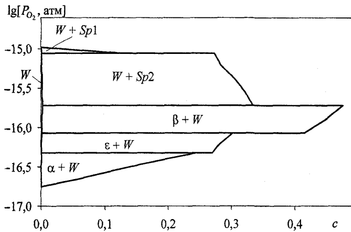
Рис. 15. Изотермическое сечение диаграммы состояния системы Fe – Ge – O при температуре 1173 К
