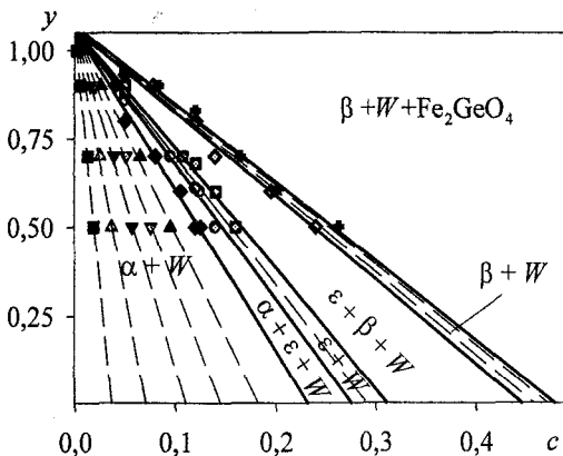
Рис. 6. Границы и коноды в областях равновесия вюститной и металлических фаз при T = 1273 \text{ K}
