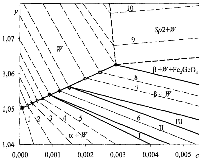
Рис. 7. Низкокислородная граница вюститной области при температуре 1273 К
