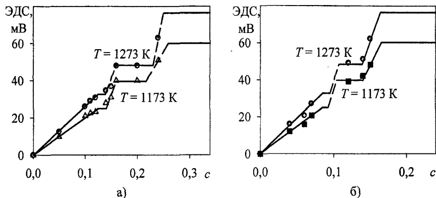
Рис. 5. Зависимость ЭДС элемента (1) от содержания германия для образцов серий \langle y = 0,5 \rangle (а) и \langle y = 0,7 \rangle (б)
