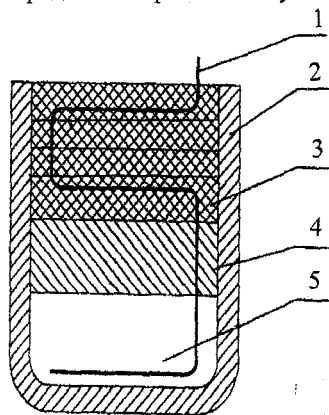
Рис. 3. Схема полужелеза
