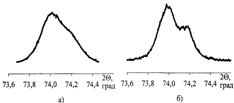
Рис. 10. Дифрактограмма закаленных образцов состава y = 1,14, c = 0,1 (а) и y = 1,2, c = 0,08 (б)
