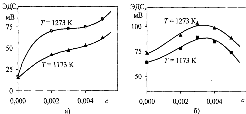
Рис. 4. Зависимость ЭДС элемента (1) от содержания германия для образцов серии \langle y = 1,06 \rangle (а) и \langle y = 1,10 \rangle (б)
