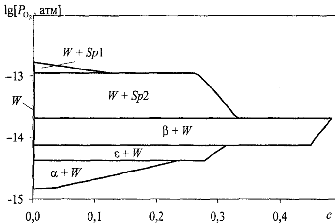
Рис. 14. Изотермическое сечение диаграммы состояния системы Fe – Ge – O при температуре 1273 К
