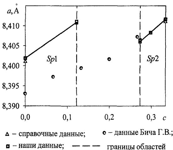
Рис. 11. Зависимость параметра решетки компонентов шпинельного раствора от его состава
