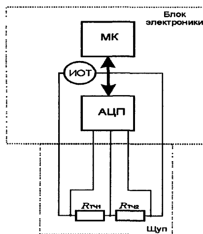
Рис. 1. Структурная схема преобразователя термосопротивления
