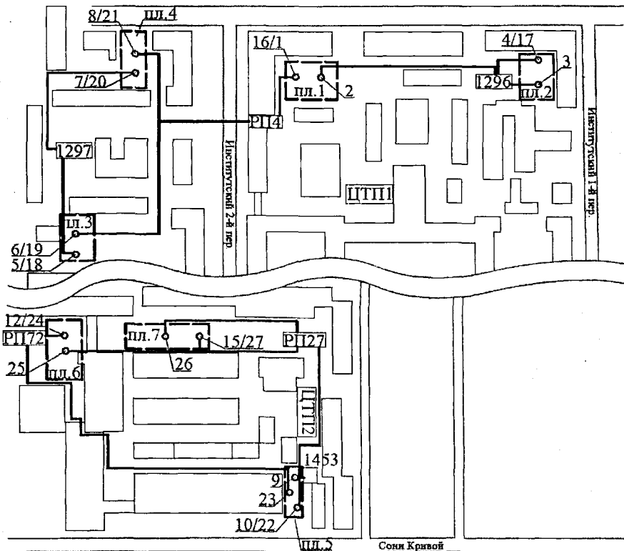
Рис. 7. План студгородка ЮУрГУ с возможными вариантами размещения РГ и трассами КЛ подключения генераторов.
