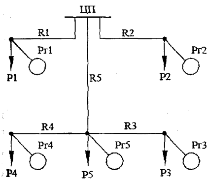
Рис. 2. Схема распределительной сети с возможными площадками для установки РГ
