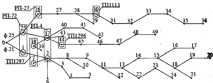
Рис. 6. Расчётная схема сети электроснабжения ЮУрГУ
