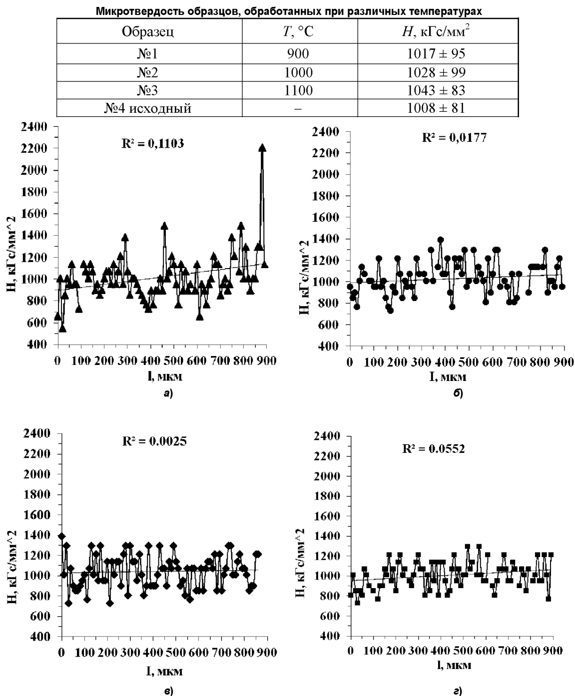
Рис. 1. Распределения микротвердости образцов, обработанных при температурах а) 900 °С, б) 1000 °С, в) 1100 °С, г) исходный
