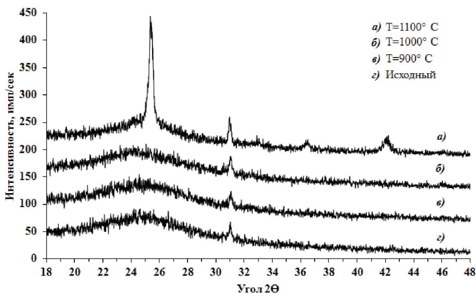
Рис. 2. График сравнения рентгенограмм исходного и термообработанных образцов
