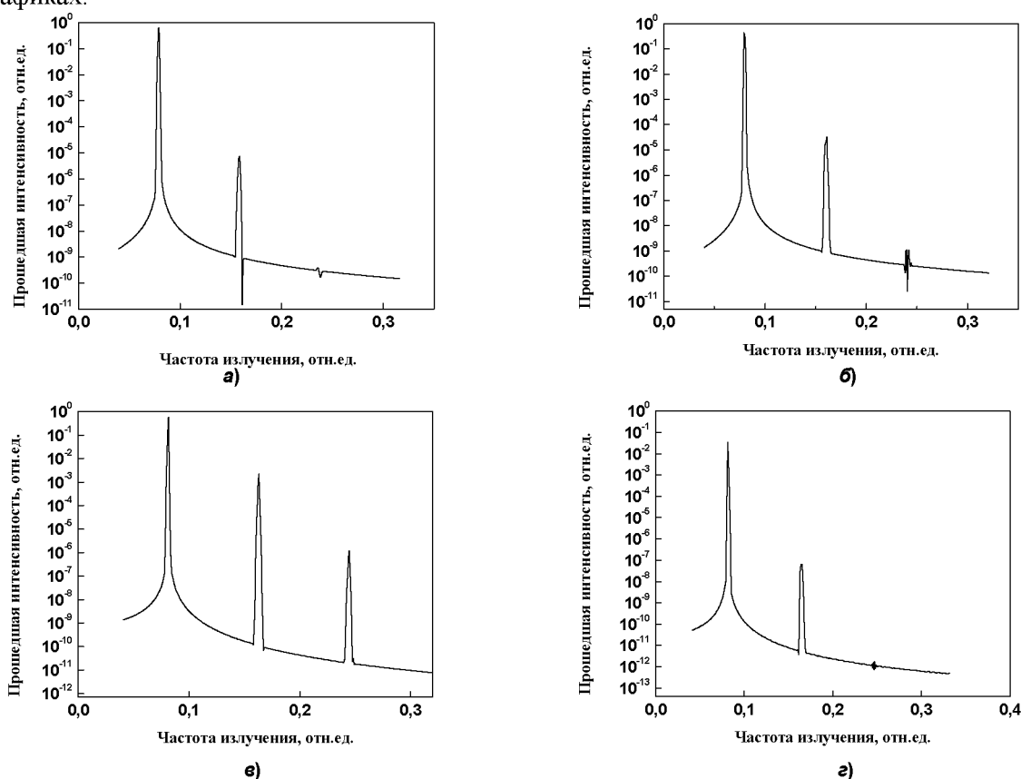
Рис. 4. ГВГ в одномерном фотонном кристалле при длине волны: а) 1266 нм, б) 1246 нм, в) 1226 нм г) 1206 нм
