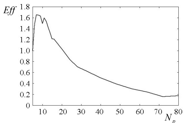
Рис. 5. Эффективность параллелизации N_{pg}=5, J=10^6 , сетка 60 \times 60 \times 60
