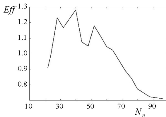
Рис. 6. Эффективность параллелизации N_{pg}=20, J=10^7 , сетка 120 \times 120 \times 60
