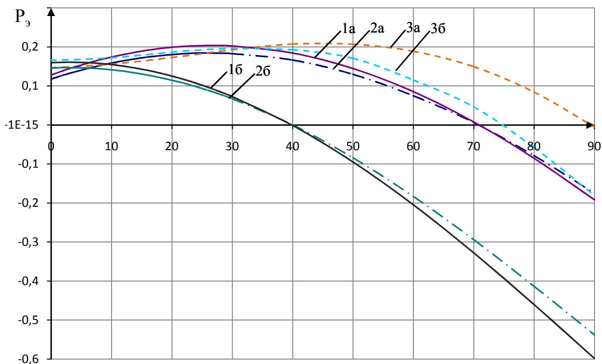
Рис. 3. Зависимость электромагнитной мощности P_e от угла коммутации \theta при \nu = 0,8 для \xi = [0,5; 0,05] , где 1а – P_e при векторном управлении для \xi = 0,5 ; 1б – для \xi = 0,05 ; 2а – P_e при 180-градусной коммутации для \xi = 0,5 ; 2б – для \xi = 0,05 ; 3а – P_e при 120-градусной коммутации для \xi = 0,5 ; 3б – для \xi = 0,05
