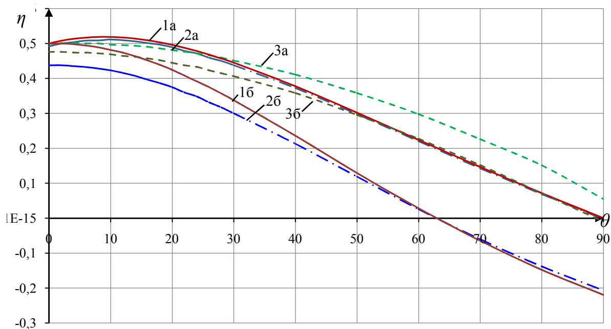
Рис. 2. Зависимость электромагнитного КПД от угла коммутации \theta при \nu = 0,5 для \xi = [0,5; 0,05] , где 1а – КПД при векторном управлении для \xi = 0,5 ; 1б – для \xi = 0,05 ; 2а – КПД при 180-градусной коммутации для \xi = 0,5 ; 2б – для \xi = 0,05 ; 3а – КПД при 120-градусной коммутации для \xi = 0,5 ; 3б – для \xi = 0,05
