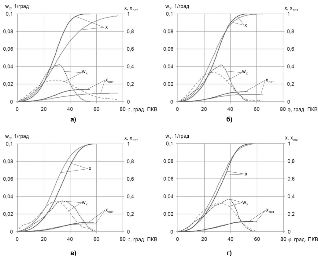
Рис. 2. Интегральные и дифференциальные характеристики выгорания топлива при работе двигателя без РОГ — — — и с РОГ — ( n = 2000 \text{ мин}^{-1} ): а – p_e = 0,35 \text{ МПа} ; б – p_e = 0,47 \text{ МПа} ; в – p_e = 0,58 \text{ МПа} ; г – p_e = 0,67 \text{ МПа}
