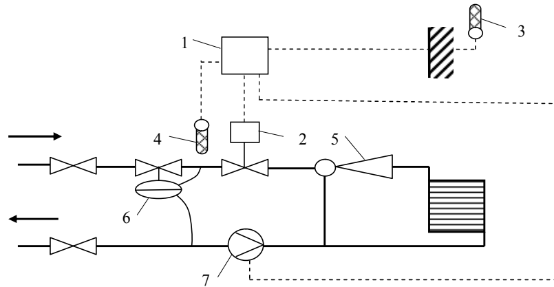
Рис. 4. Схема 2-го варианта импульсной системы управления: обозначения как на рис. 3
