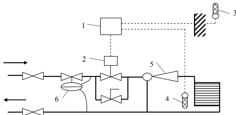
Рис. 1. Схема двухпозиционной САР: 1 – контроллер, 2 – двухходовой клапан с электроприводом и байпасной линией, 3 – датчик температуры наружного воздуха, 4 – датчик температуры обратной воды, 5 – элеватор, 6 – регулятор перепада давления
