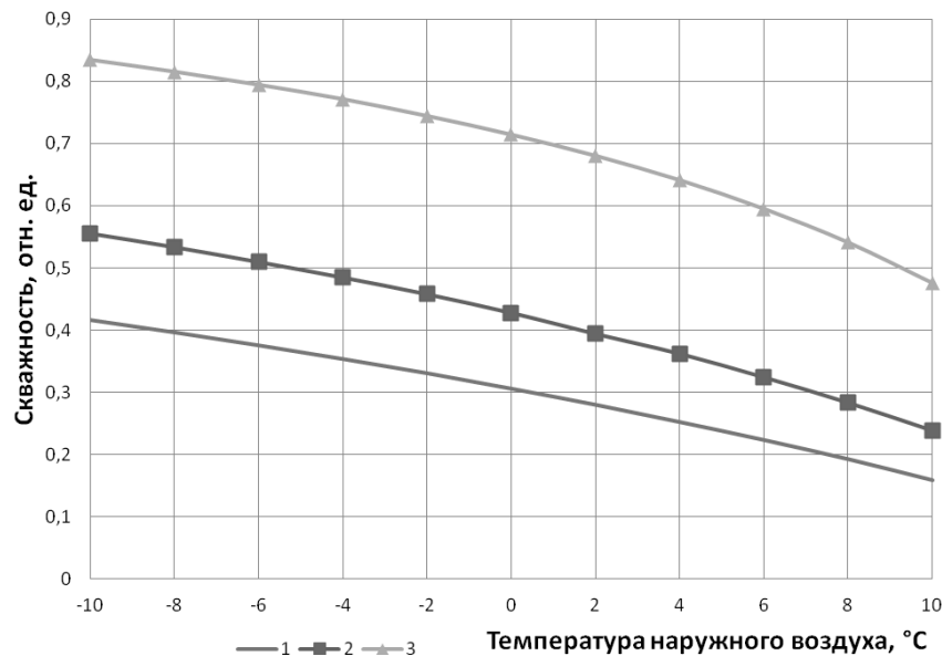
Рис. 2. Зависимость скважности управляющих импульсов \gamma от температуры наружного воздуха t_H
