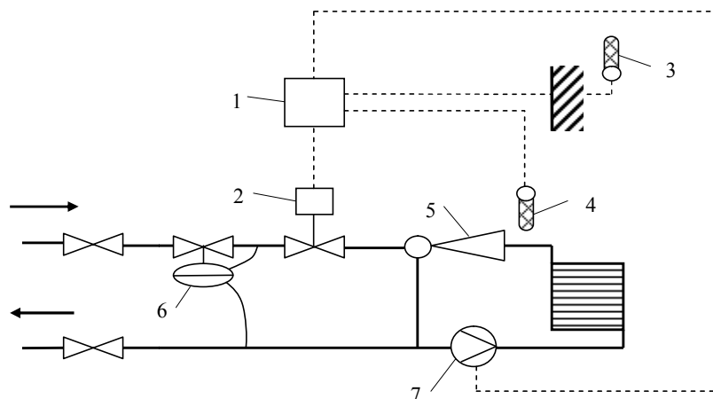
Рис. 3. Схема 1-го варианта импульсной системы управления: 1–6 – обозначения как на рис. 1; 7 – расходомер
