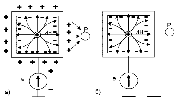
Электростатическое экранирование
