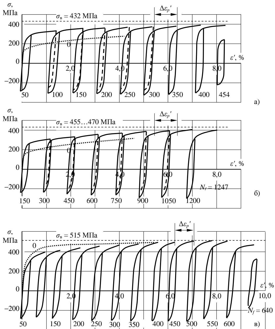
Рис. 2. Блочное нагружение (кривая 0 – статическое нагружение): а) сплав ЭП864, 600 °С; \Delta\varepsilon_p'' = 1,06\% ,
