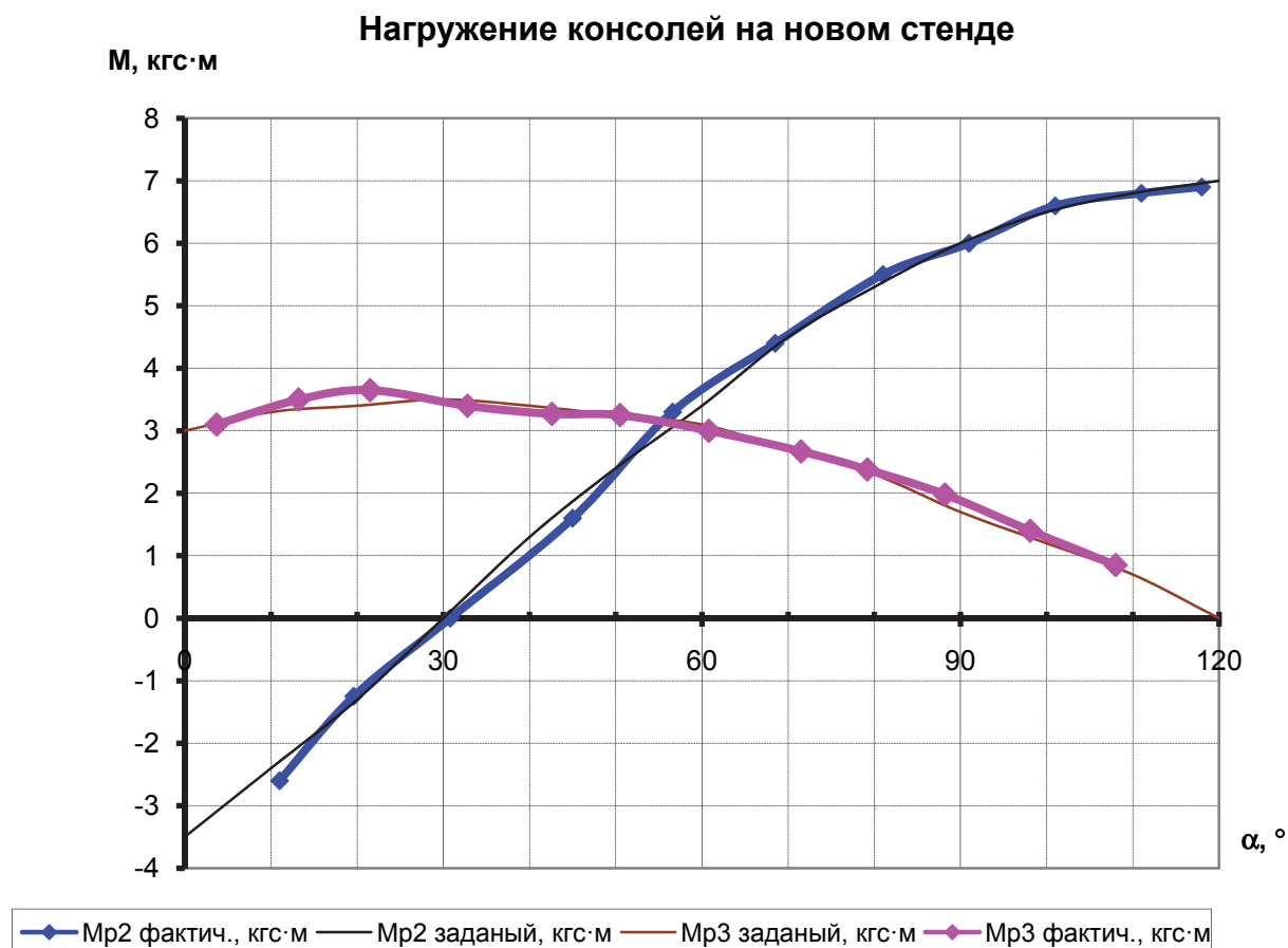
Рис. 10. График зависимости моментов от угла поворота консоли
