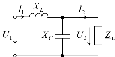
Рис. 1. Схема LC-фильтра
