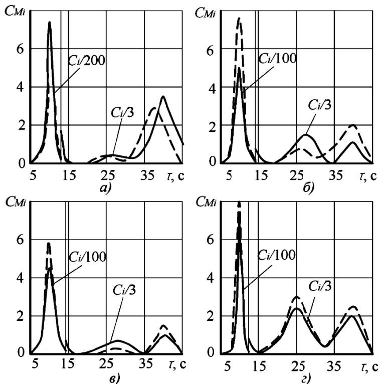
Рис. 2. Хроматограммы содержания компонентов в продуктах распада при электроразряде: а – октан; б – дизельное топливо ДЛ ГОСТ 4749-78; в – бензин А-76; г – спирт этиловый; ———— – 3 кВ, - - - - - 2 кВ [6]
