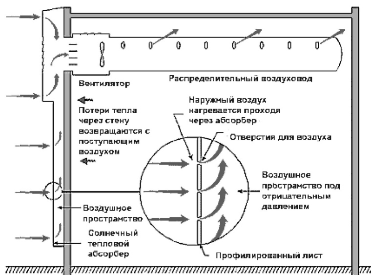
Рис. 3. Схема воздушного коллектора
