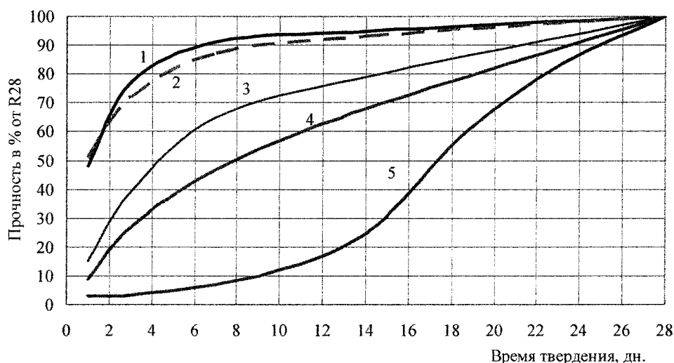
Рис. 1. Кривые кинетики твердения бетонов на различных видах вяжущего: 1 – шлакощелочной бетон (состав вяжущего: шлак нейтральный, щелочной компонент метосиликат натрия), 2 – бетон на глинозёмном цементе марки 200, 3 – бетон на шлакопортландцементе марки 400, 4 – бетон на портландцементе марки 250, 5 – шлакощелочной бетон (состав вяжущего: шлак кислый, щелочной компонент сода кальцинированная)
