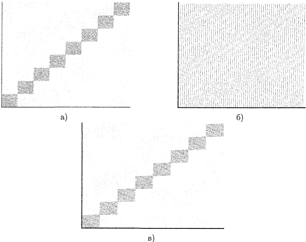
Рис. 3. а) профиль обращений в память к массиву А; б) профиль обращений в память к массиву В; в) профиль обращений в память к массиву С
