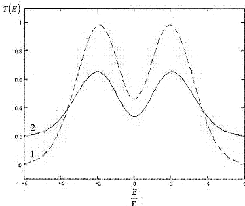
Туннельная прозрачность гетеробарьера \text{EuS}
