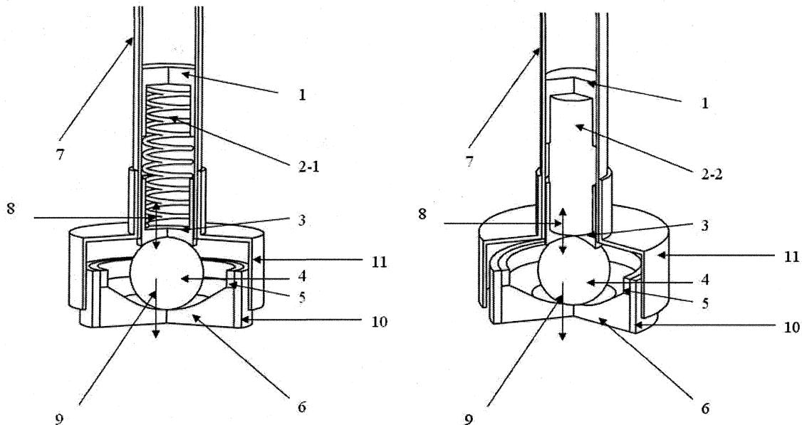
Рис. 2. Варианты виброгасителей
