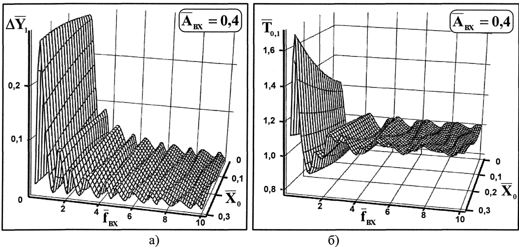
Рис. 2. Пространства динамического состояния \Delta\bar{Y}_1, \bar{T}_{0,1} = f(\bar{X}_0, \bar{f}_{BX})
