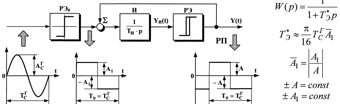
Рис. 8. Комбинированное интегрирующее УС «компаратор – РП» с частичной адаптацией
