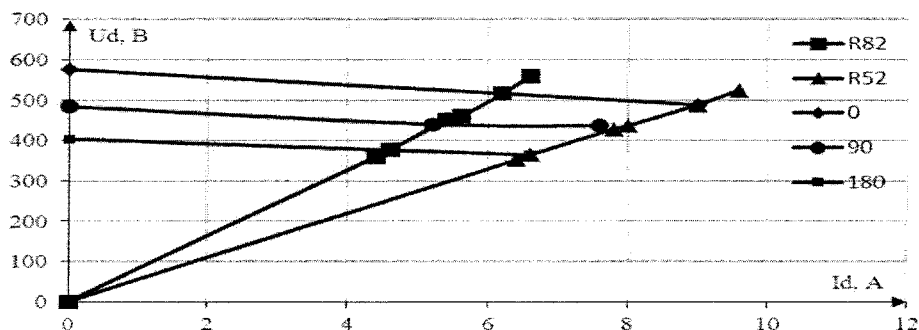
Рис. 5. Характеристика компенсированного выпрямителя при фазовом регулировании (амплитудное напряжение АИН Uaин=300 В)
